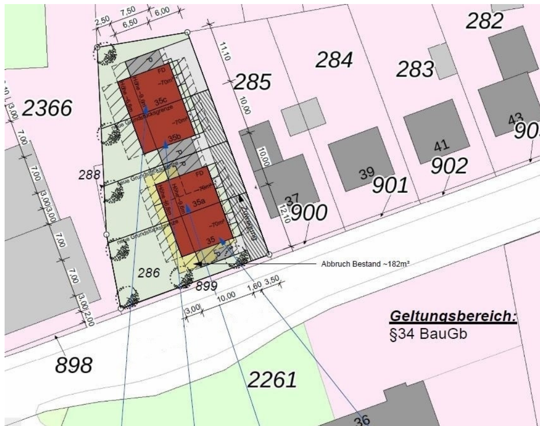
Lageplan - 2 Doppelhäuser
